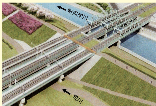
荒川橋梁部周辺の堤防かさ上げ工事
